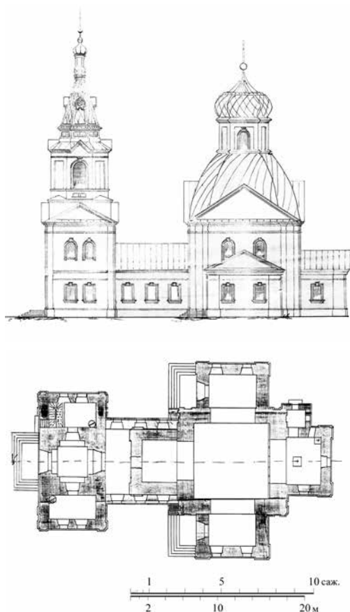
Рис. 43. Креслення Георгіївської церкви с. Ковчина.
