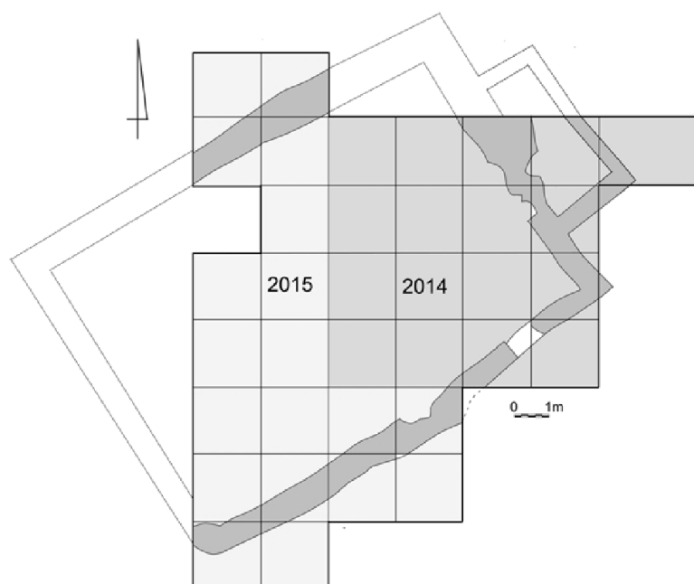
Рис. 6. План підмурків церкви Іоакима та Анни, досліджених у 2013–2015 рр.
