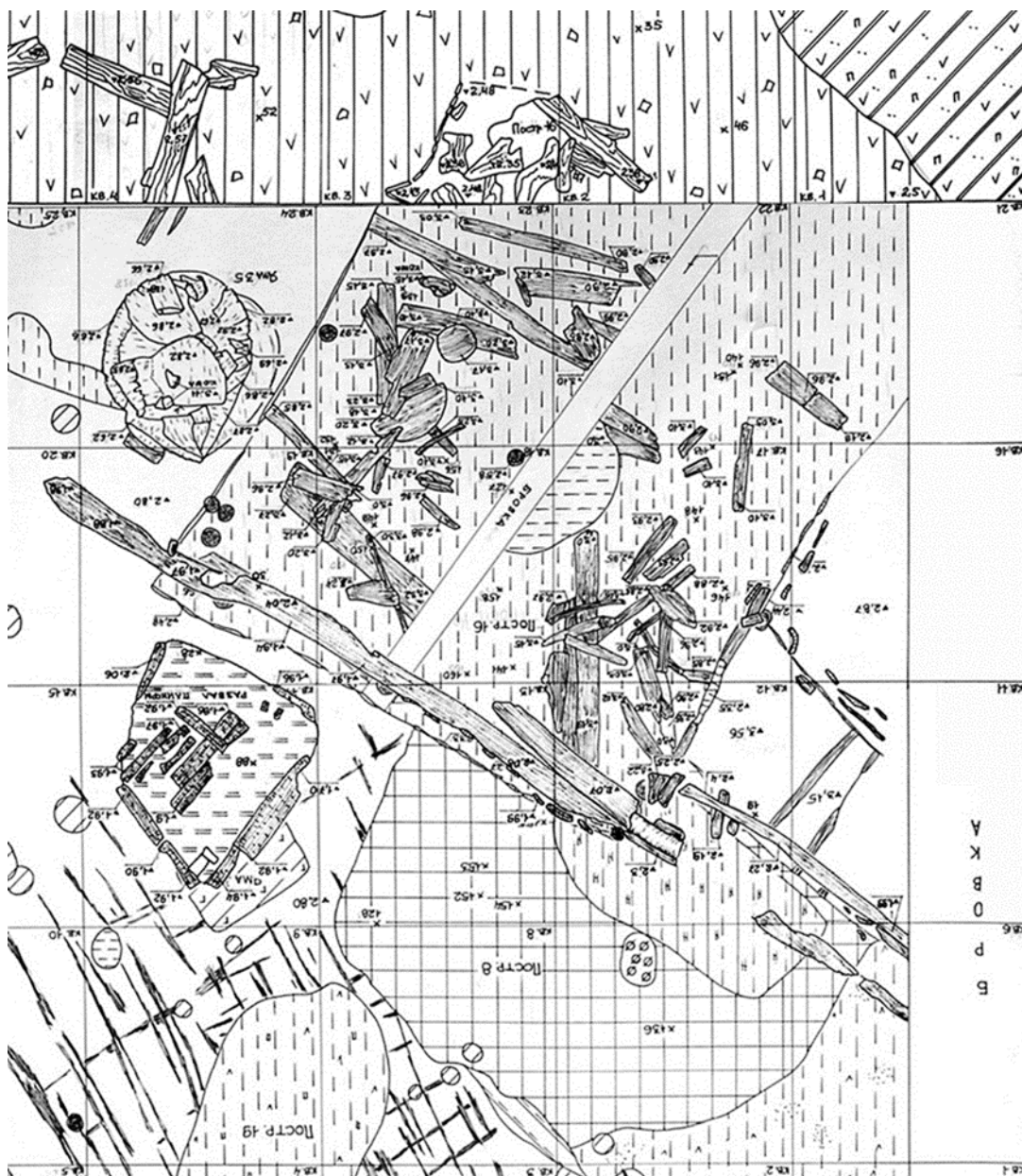
Рис. 1. План постройки № 16 на уровне зафиксированных верхних деревянных конструкций
