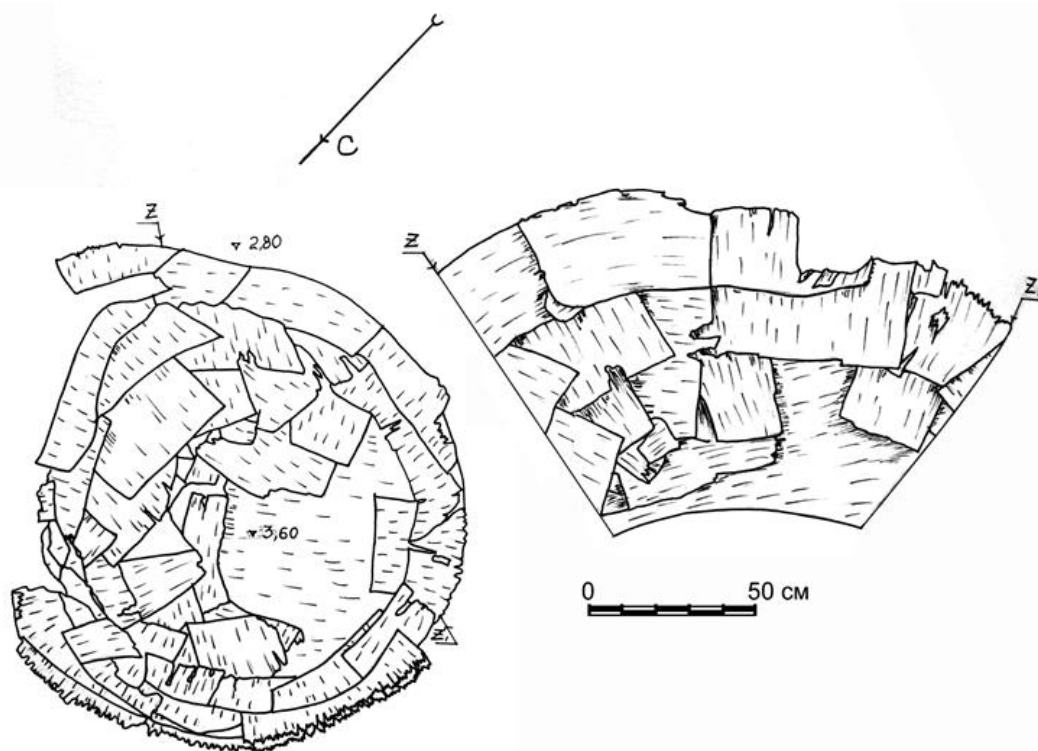
Рис. 7. План бересты в яме № 35
