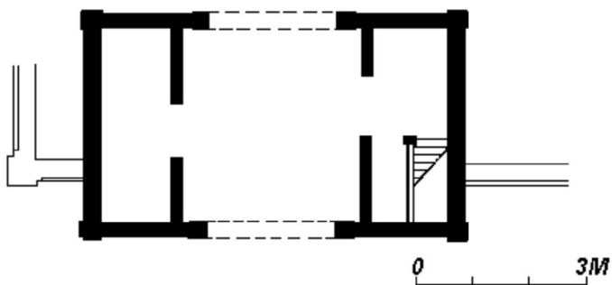
Рис. 14. Надбрамна башта монастиря в Низкиничях, фото та план [за: Пам'ятники градостроїтельства УССР. К., 1985. Т.2. С. 71].
