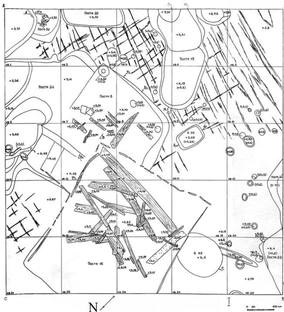
Рис. 3. Планы заполнения и конструкции подклетов построек №№ 8, 16
