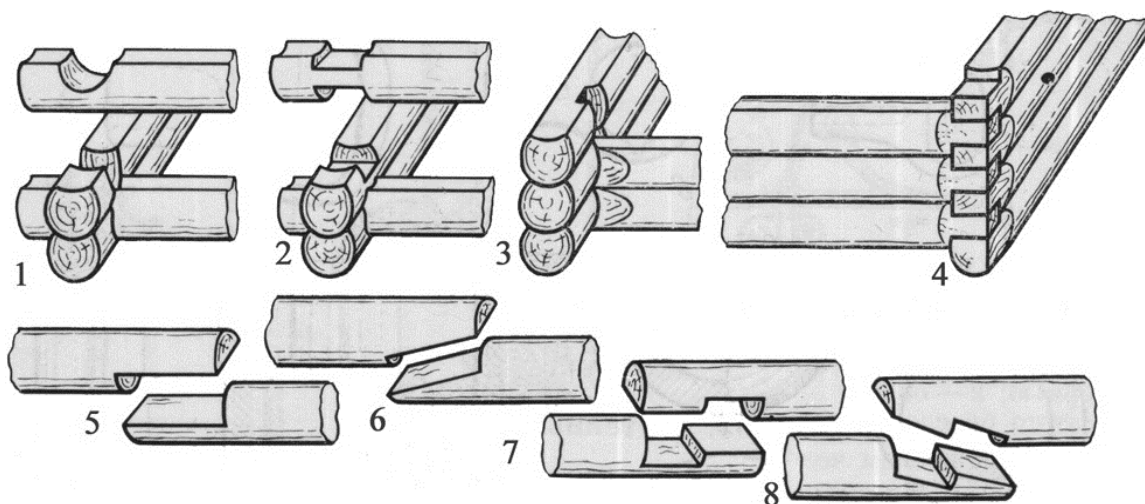
Рис. 5. Зразки дерев'яних з'єднань (за Б.О. Колчиним [1985, табл. 103])
